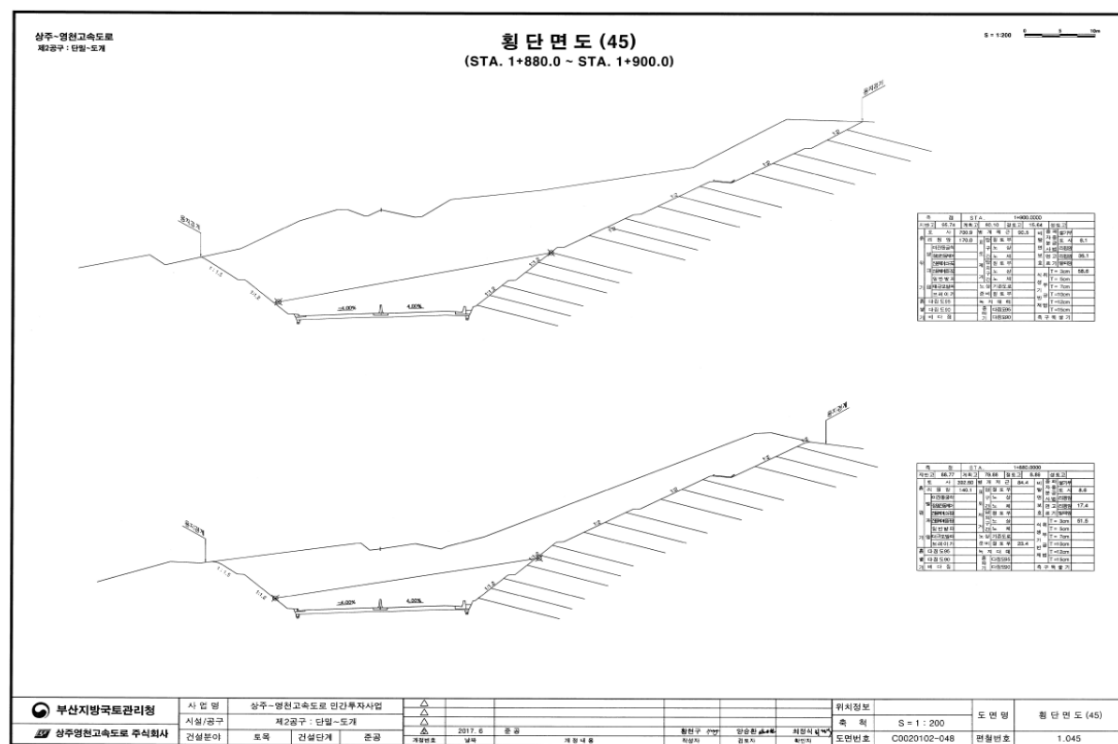
【그림 6.4】 표준횡단면도
